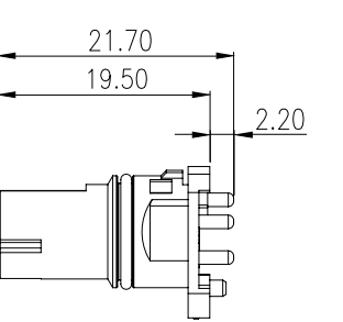
母端插座
