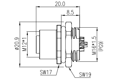
母端插座
