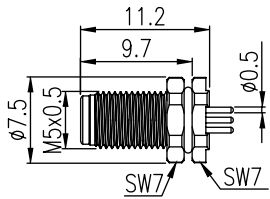
公端插座
