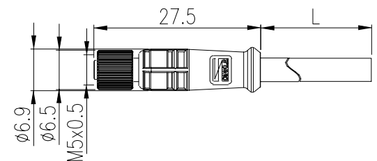
单边 180° 母端
