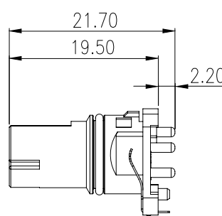
母端插座
