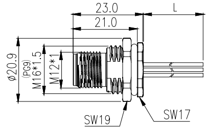
公端插座
