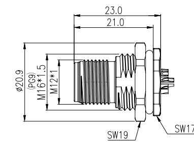
公端插座
