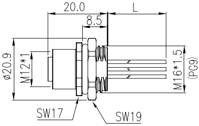
母端插座
