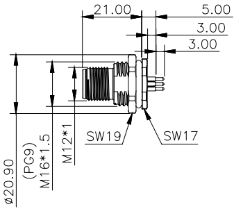
公端插座
