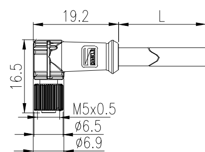
单边 90° 母端
