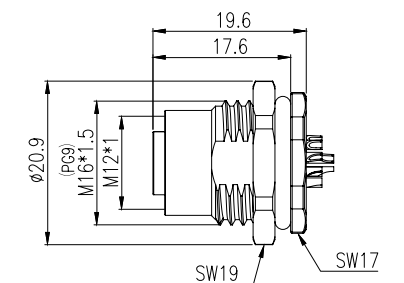
母端插座
