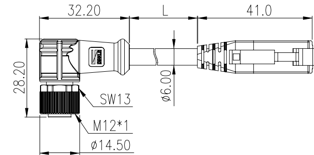
90° 母端 +RJ45
