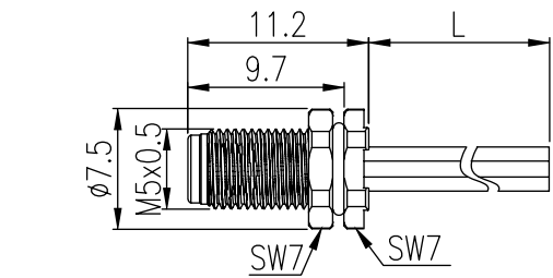
公端插座
