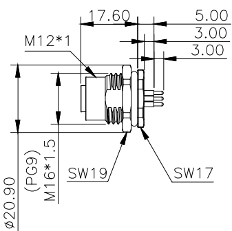
母端插座
