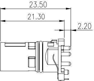
公端插座
