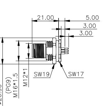
公端插座
