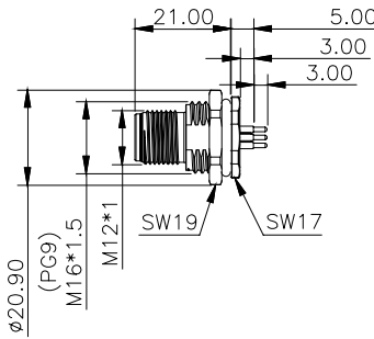
公端插座
