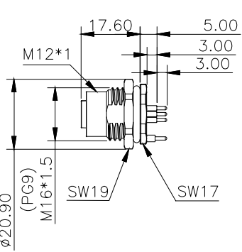
母端插座
