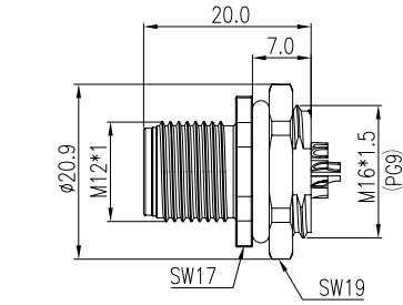
公端插座
