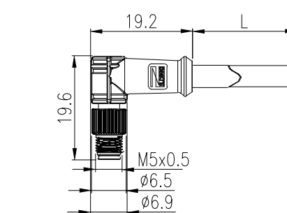
单边 90° 公端
