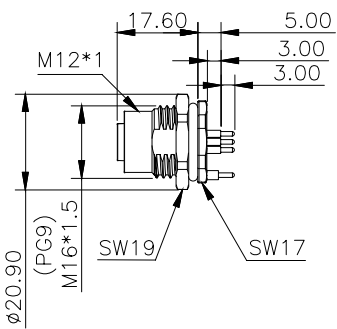
母端插座
