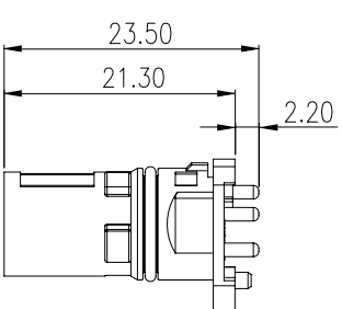
公端插座
